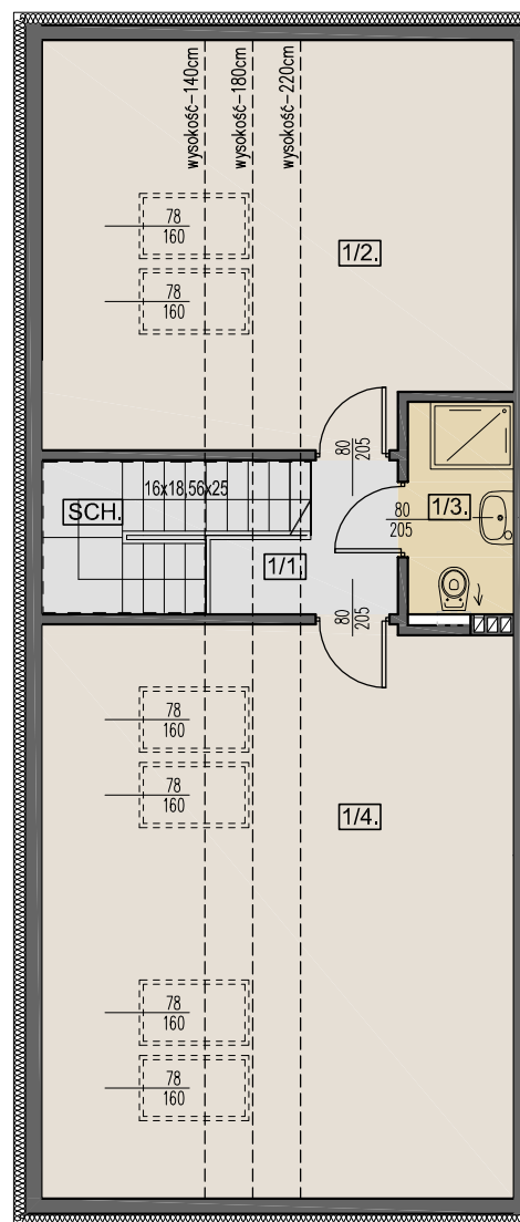
RZUT PODDASZA
