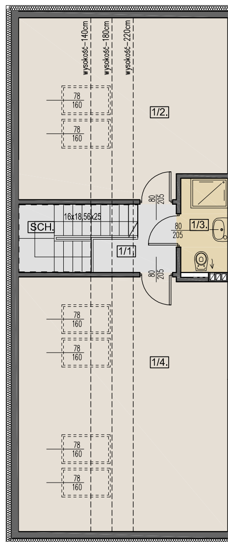
RZUT PODDASZA
