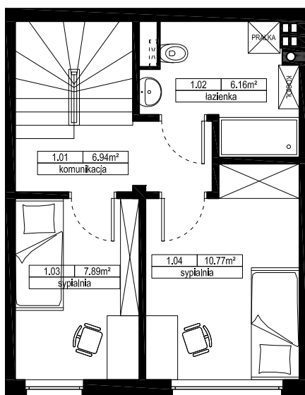
RZUT I PIĘTRA
